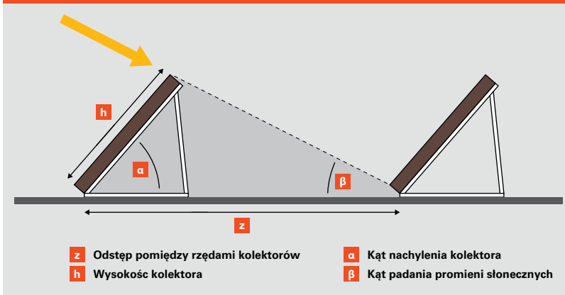
Rys. B.1.6-11 Odległość między rzędami kolektorów
