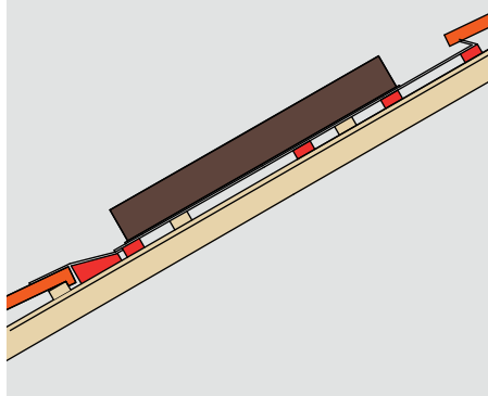
Rys. B.1.6-7 Montaż w połaci dachu (przekrój)
