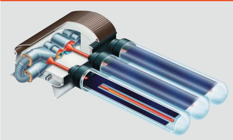
Przekrój kolektora próżniowego typu Heatpipe
