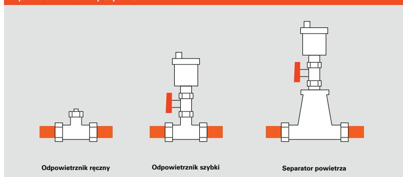
Rys. B.3.3-1 Warianty odpowietrzników
