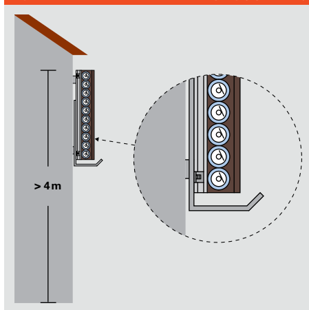
Rys. B.1.6–15 Montaż na fasadzie w pozycji pionowej
