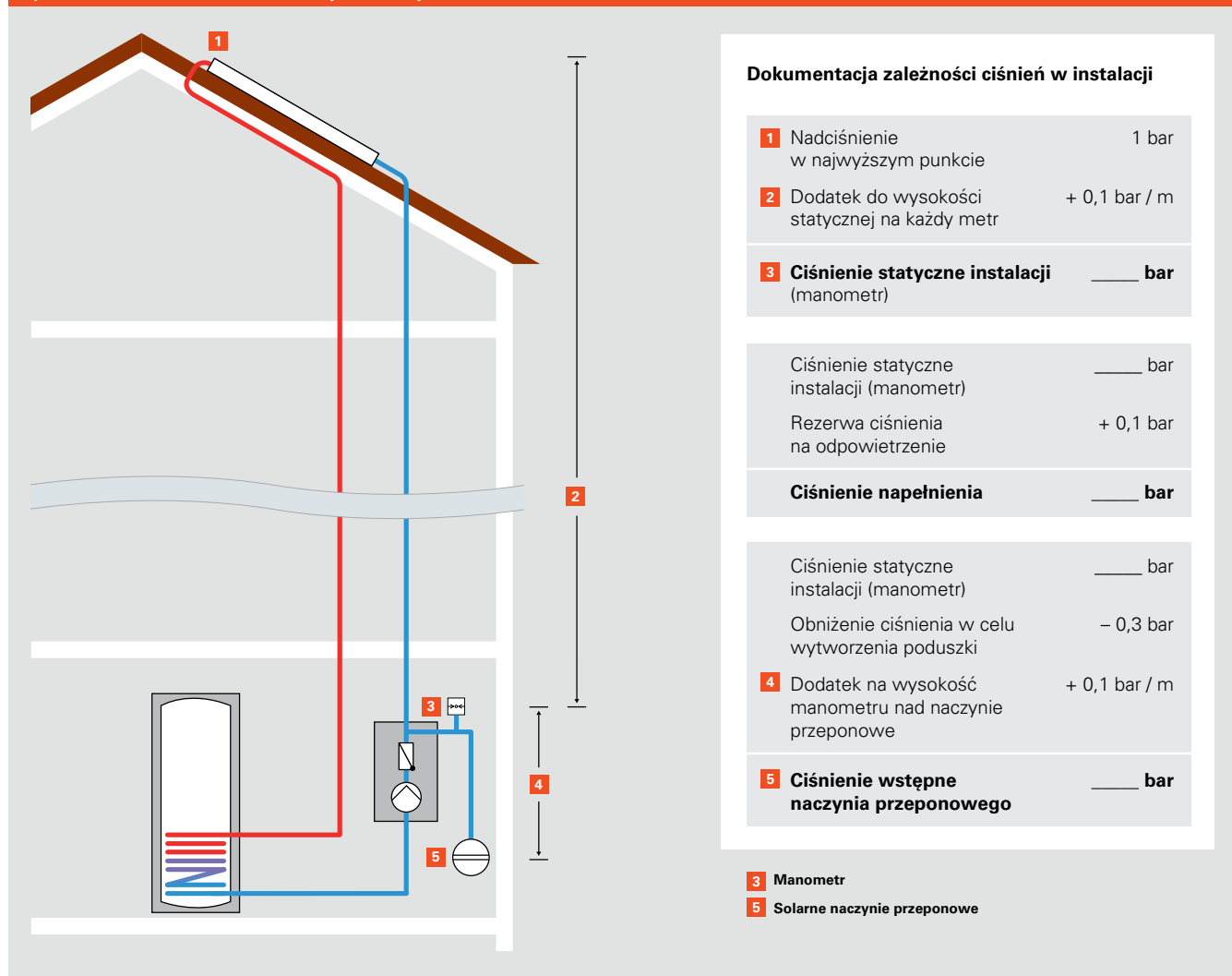
Rys. E.1.1-3 Zależność ciśnień w instalacji słonecznej
