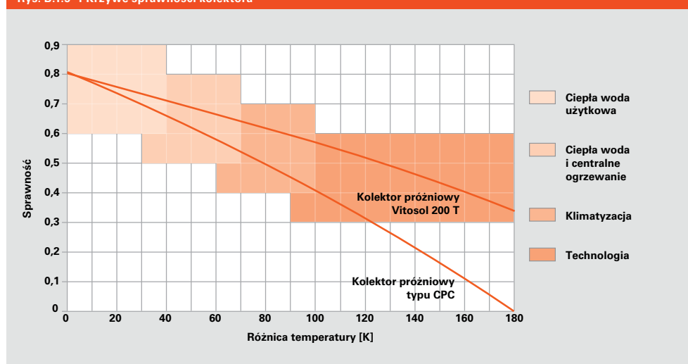
Rys. B.1.5-1 Krzywe sprawności kolektora
