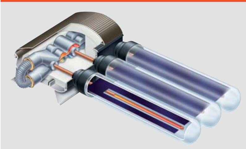
Przekrój kolektora próżniowego z suchym połączeniem rur heatpipe
