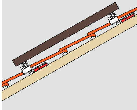
Rys. B.1.6-5 Montaż na dachu (przekrój)
