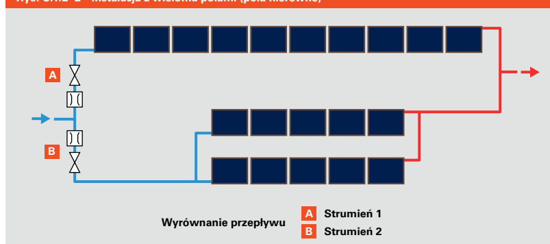
Rys. C.1.2-2 Instalacja z wieloma polami (pola nierówne)
