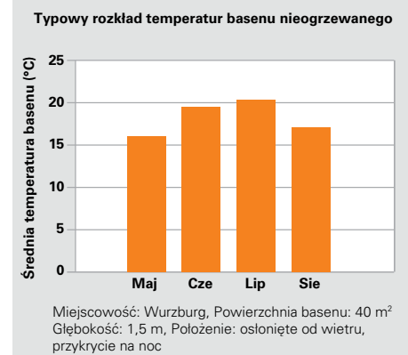
Rys. C.2.4-1 Temperatury basenu otwartego
