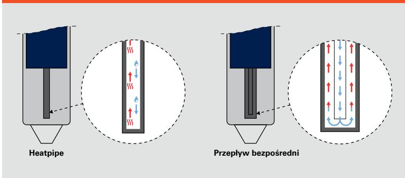
Rys. B.1.2-4 Absorber Heatpipe z bezpośrednim przepływem
