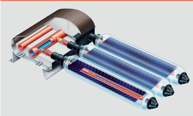
Przekrój kolektora próżniowego z przepływem bezpośrednim
