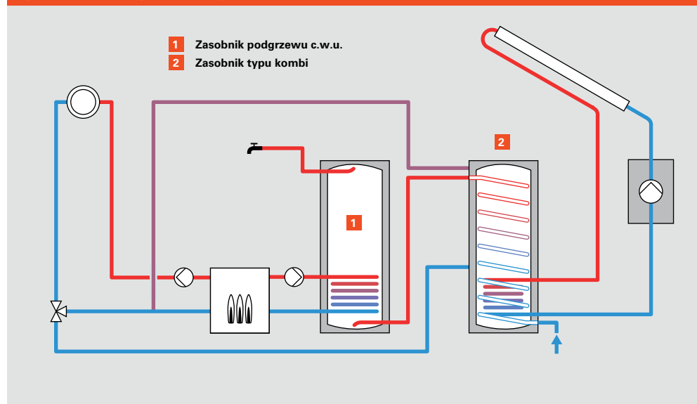
Rys. C.2.2-5 Instalacja z dodatkowym zasobnikiem
