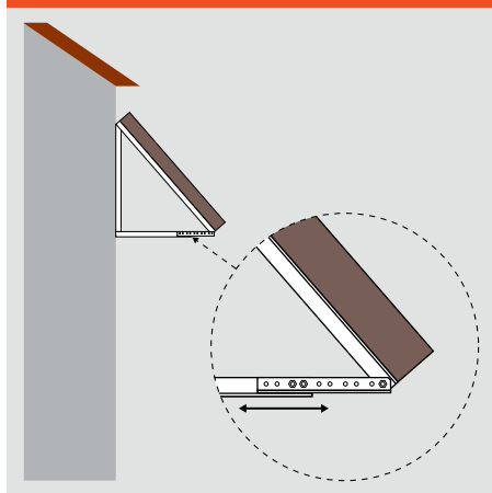
Rys. B.1.6–16 Montaż ukośny na fasadzie
